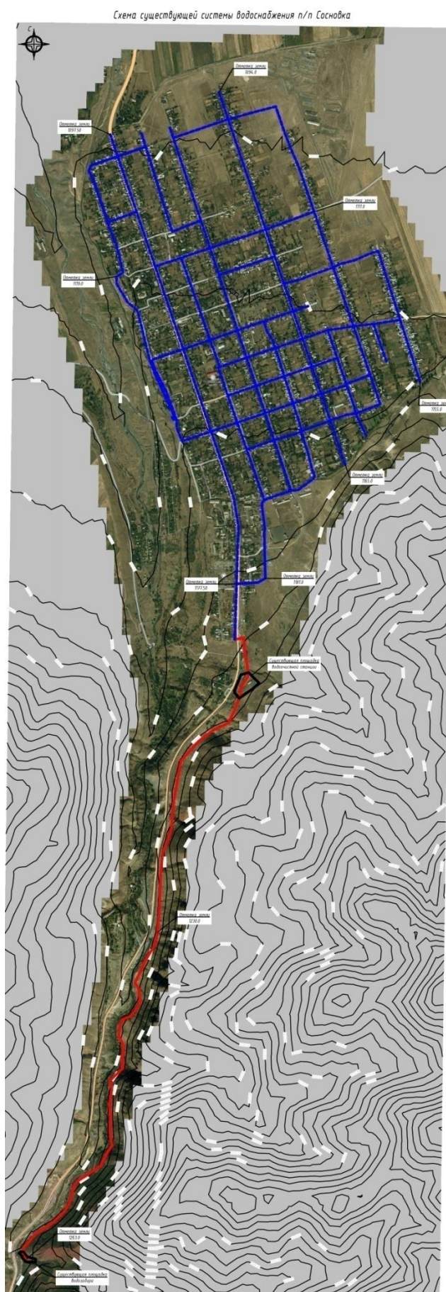
Схема существующей системы водоснабжения п/п Сосновка
